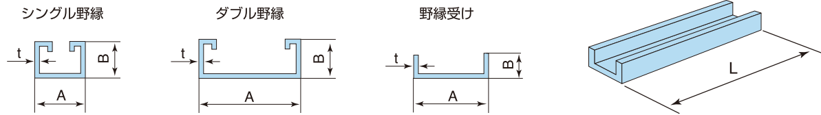
【表 4】天井下地材の構成部材の寸法
